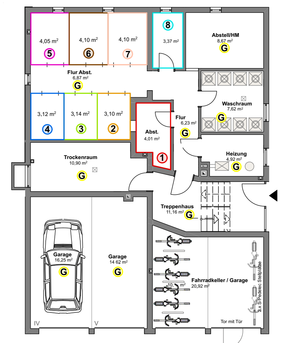
Grundriss Kellergeschoss
