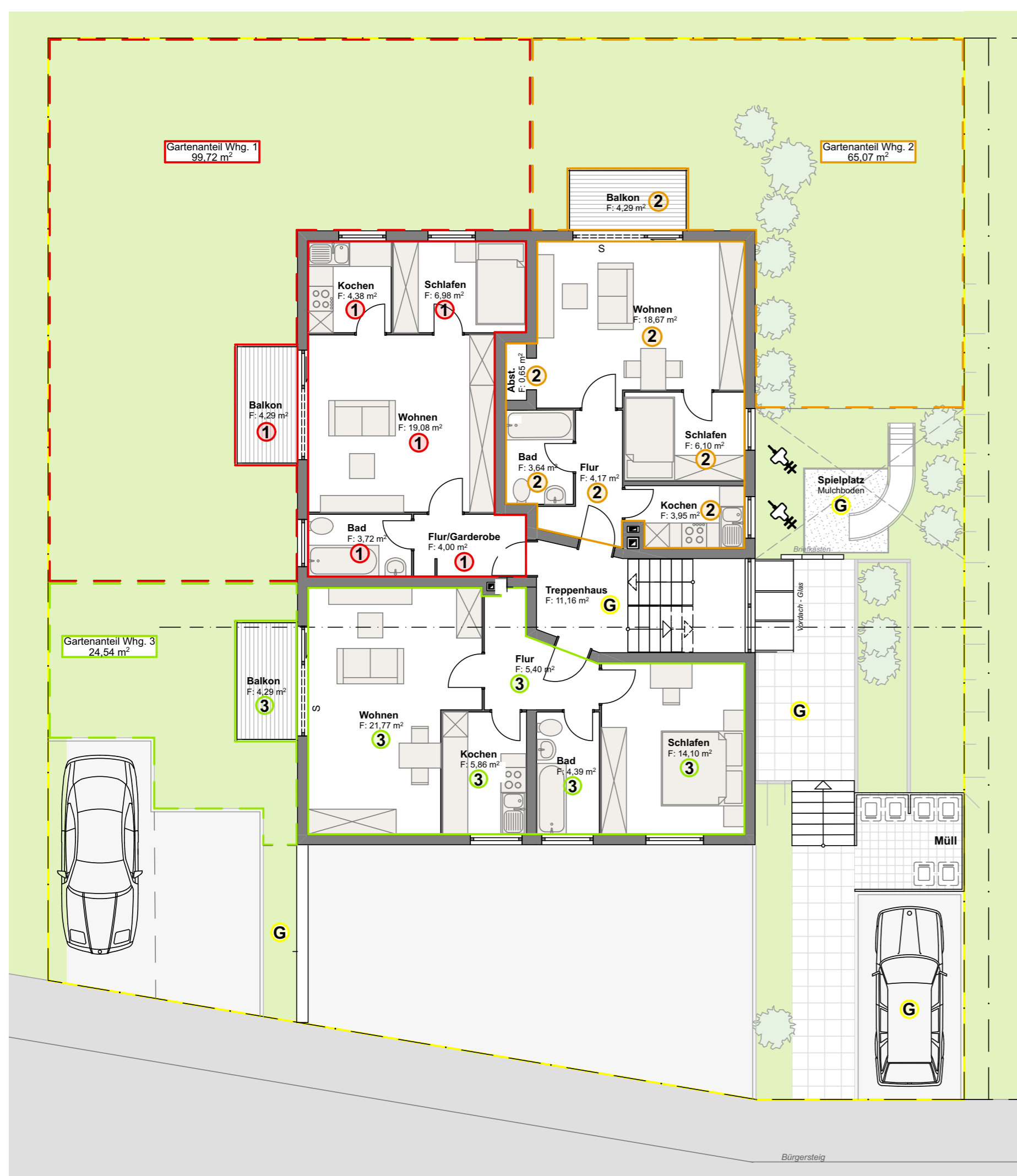
Grundriss Erdgeschoss mit Gartenanteilen
